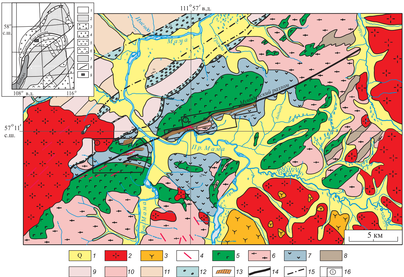
Рис. 1. Геологическая карта золоторудного поля Мукодек (составлена с использованием материалов геолого-поисковых работ 2008 и 2012 гг.)
