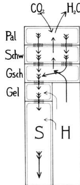
Fig. 22. Saftströmungen im assimilierenden Blatt, Ergänzung zum Schema Fig. 10 u. 12. Pal Palisadenparenchym, Schw Schwammparenchym, Gsch Gefäßbündelscheide, Gel Geleitzelle, S Siebröhre, H Holzbahn (Hydrom). Ungefiederte Pfeile: Wasser; einfach gefiederte Pfeile: \text{CO}_2 ; doppelt gefiederte Pfeile: Lösung der Assimilate. Entsprechend der Abnahme der Strömungswiderstände strömt im Gefäßbündel Wasser aus dem Hydrom ins Leptom.
